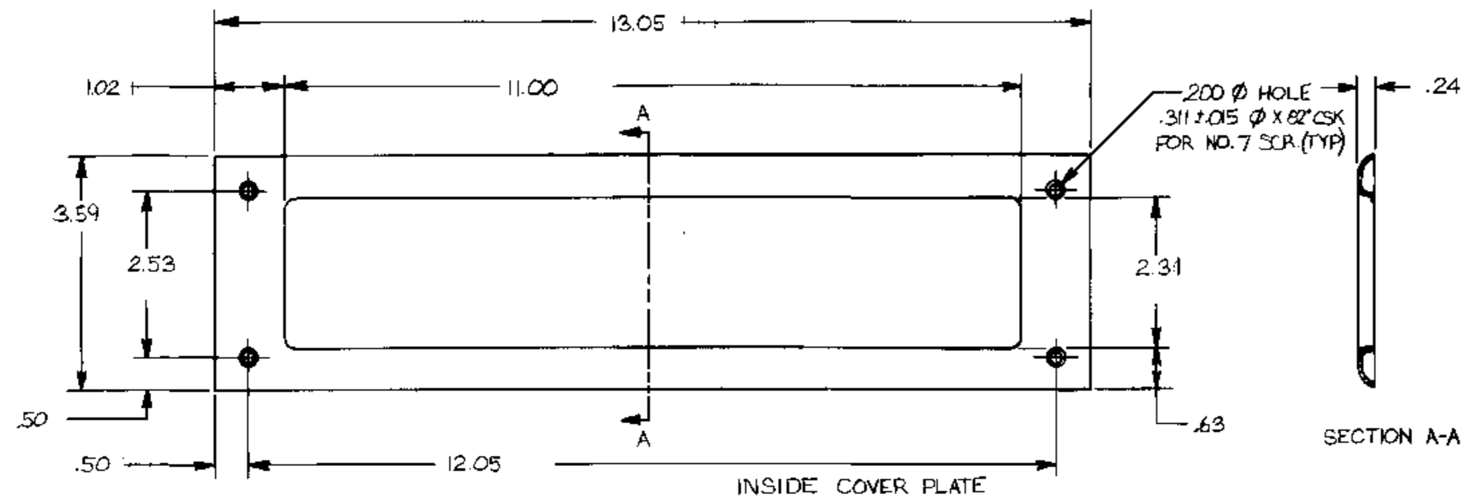
2X11 TEMPLATE
